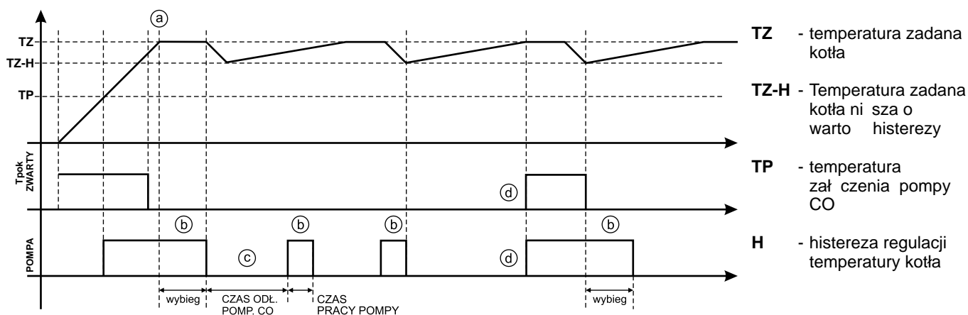
Rys.8. Zmiany temperatury na kotle i zachowanie urz dze dla ALGORYTM=2
