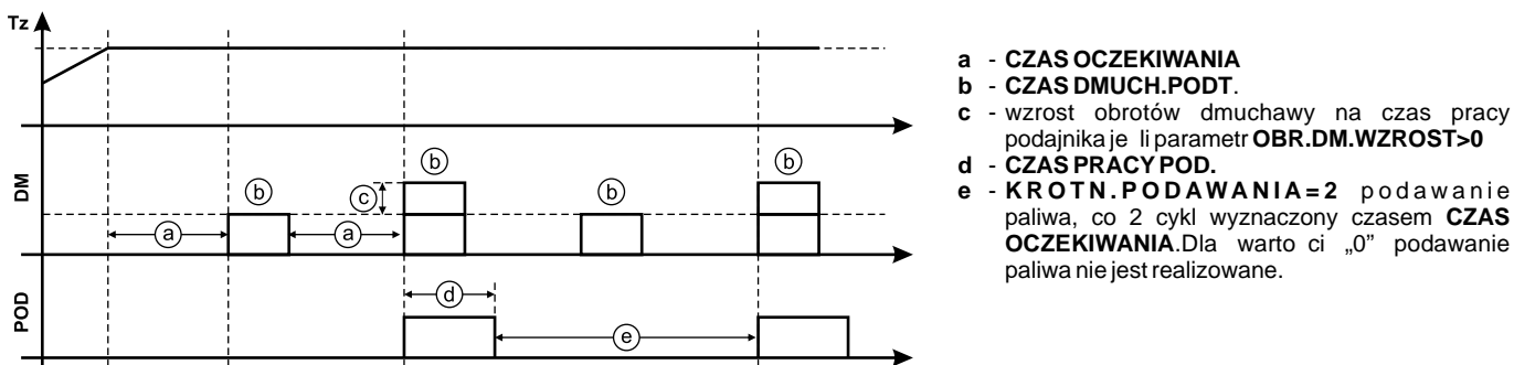
Rys.13. Interpretacja graficzna sposobu działania podajnika i dmuchawy.
