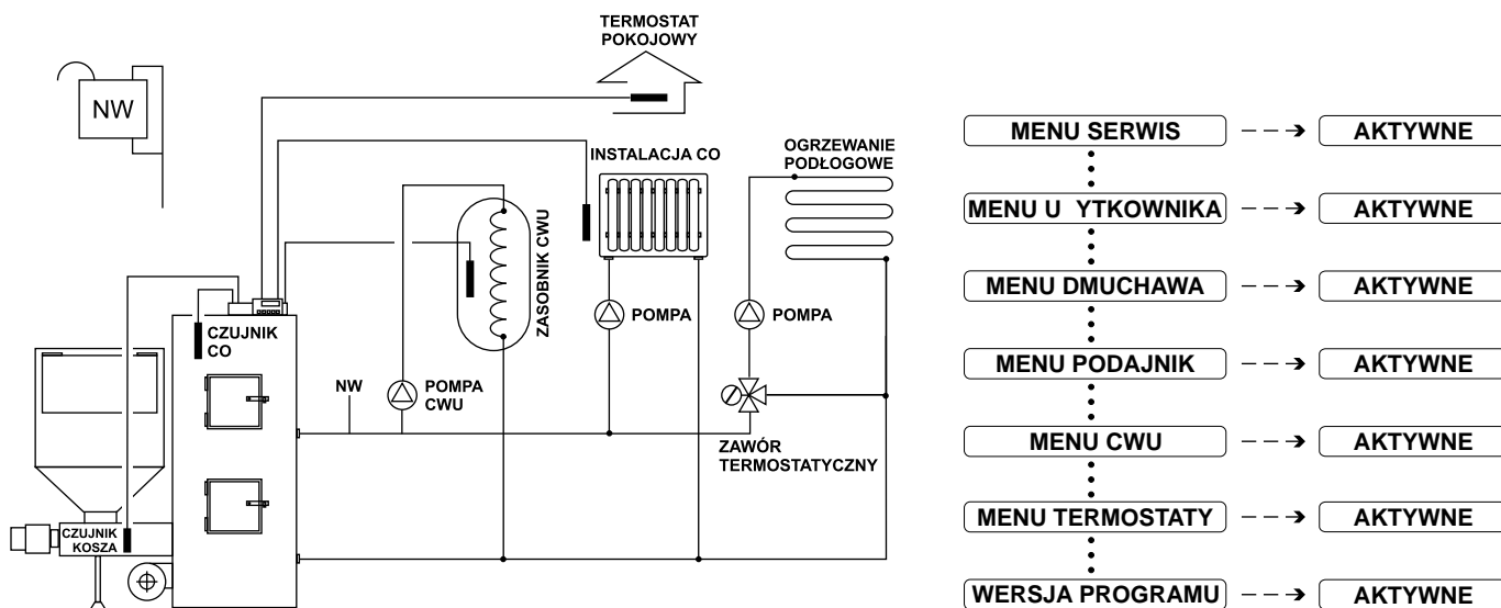
Rys.4. Sterowanie kotłem podajnikowym z jednym obiegiem grzewczym sterowanym pomp w funkcji termostatu pokojowego, ogrzewaniem podłogowym sterowanym zaworem termostatycznym, zasobnikiem ciepłej wody.
