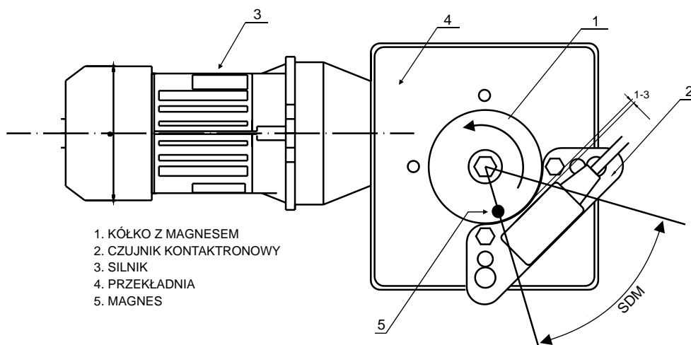
Rys.9. Mocowanie kontaktronu do przekładni.
