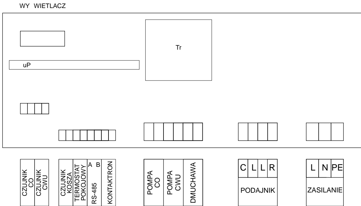
Rys.16. Widok płyty głównej z kostkami montażowymi do podłączenia urządzeń wejściowych/wyjściowych.
