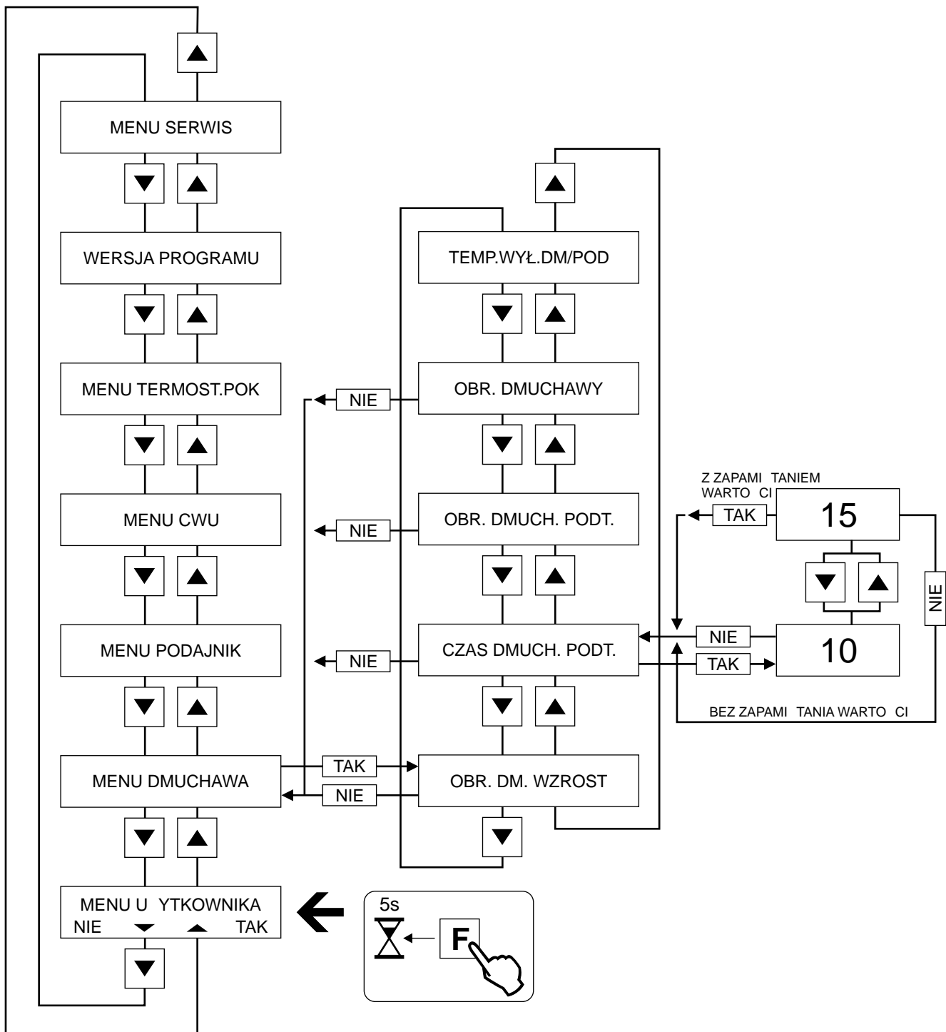
Rys.6. Przykładowe poruszanie się po menu w celu zmiany parametrów
