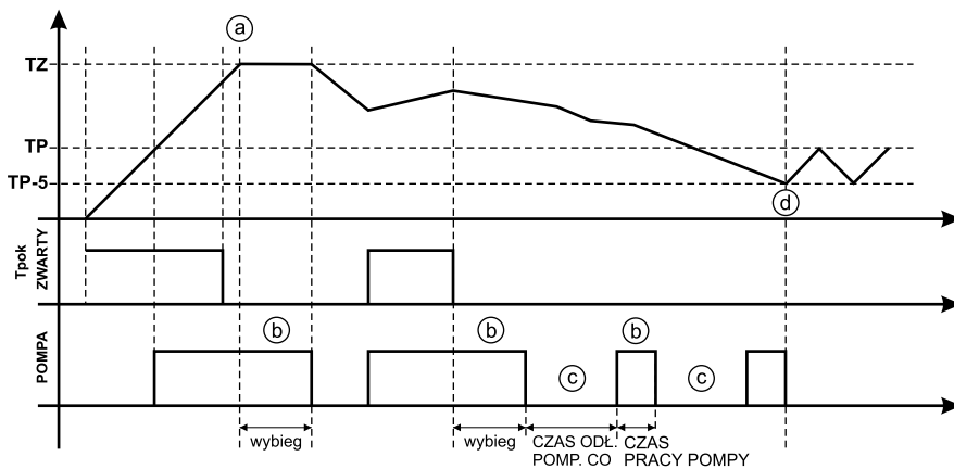
Rys.7. Zachowanie modułu i przebieg temperatury na kotle dla ALGORYTM=0
