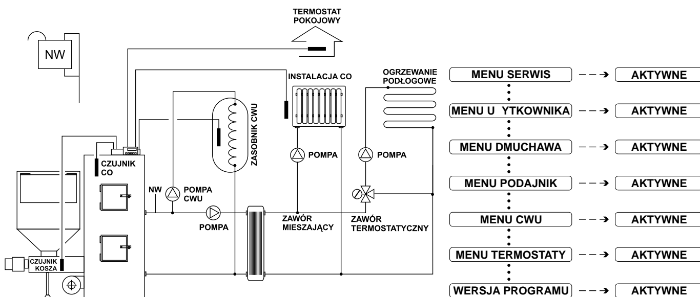
Rys.5. Sterowanie kotłem podajnikowym z jednym obiegiem grzewczym sterowanym pomp w funkcji termostatu pokojowego, ogrzewaniem podłogowym sterowanym zaworem termostatycznym, zasobnikiem ciepłej wody. Wymiennik płytowy do rozdzielenia układu otwartego i zamkniętego.
