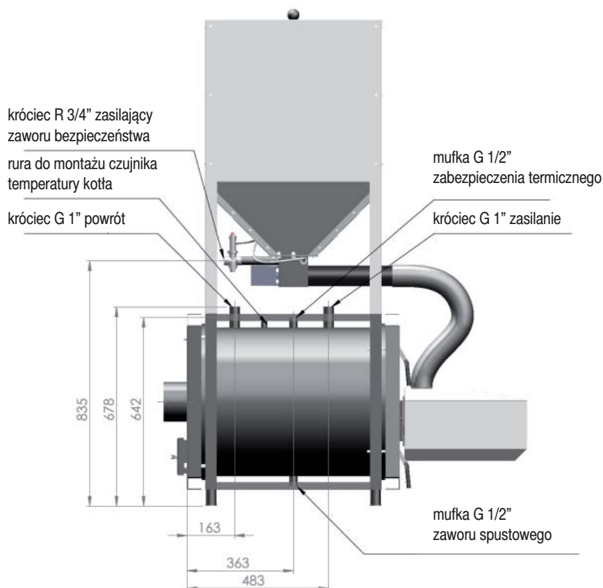
Rys. 02. Rozmieszczenie i wymiary króćców przyłączeniowych.
