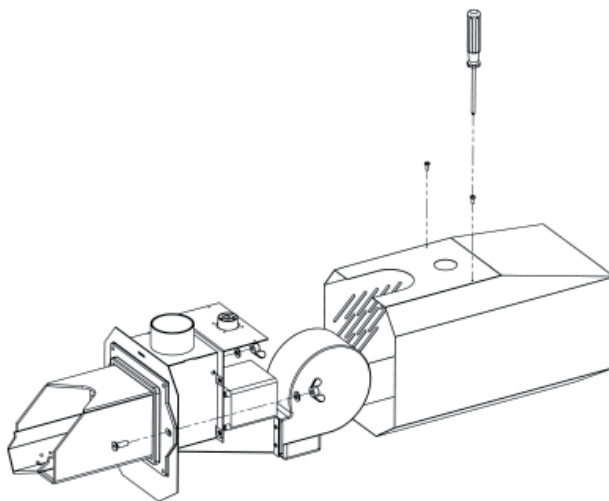
Rys. 04. Demontaż obudowy palnika Platinum Bio
