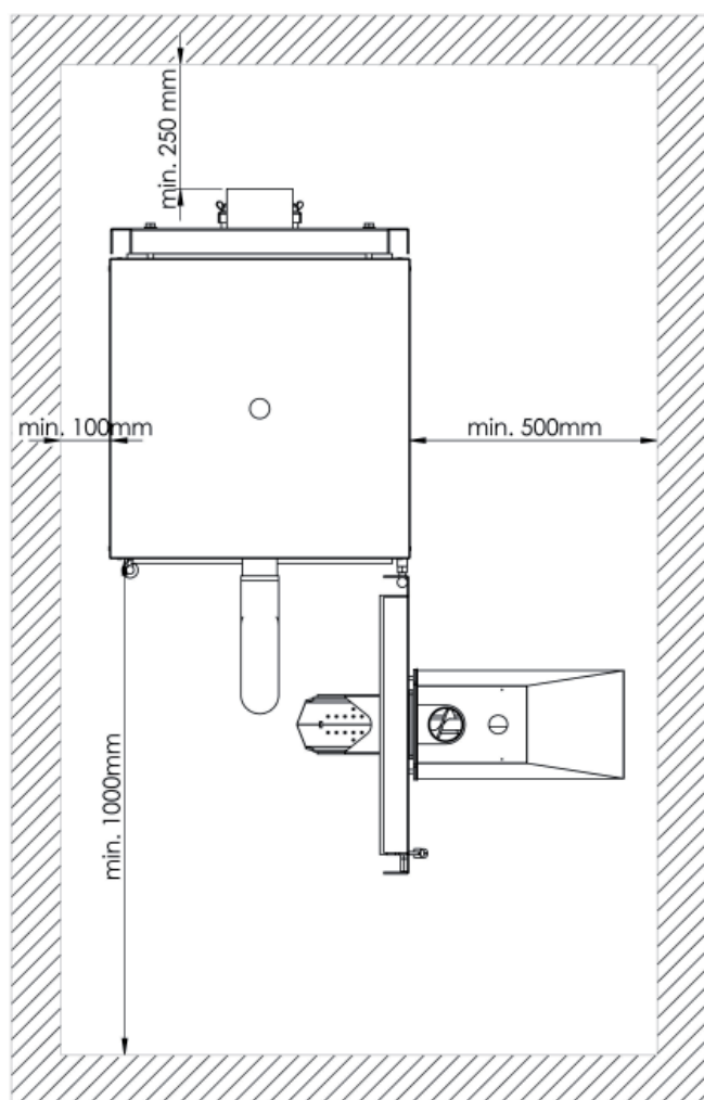
Rys. 03. Ustawienie kotła w kotłowni.
