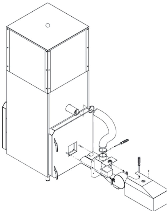
Rys. 05. Montaż palnika Platinum Bio
