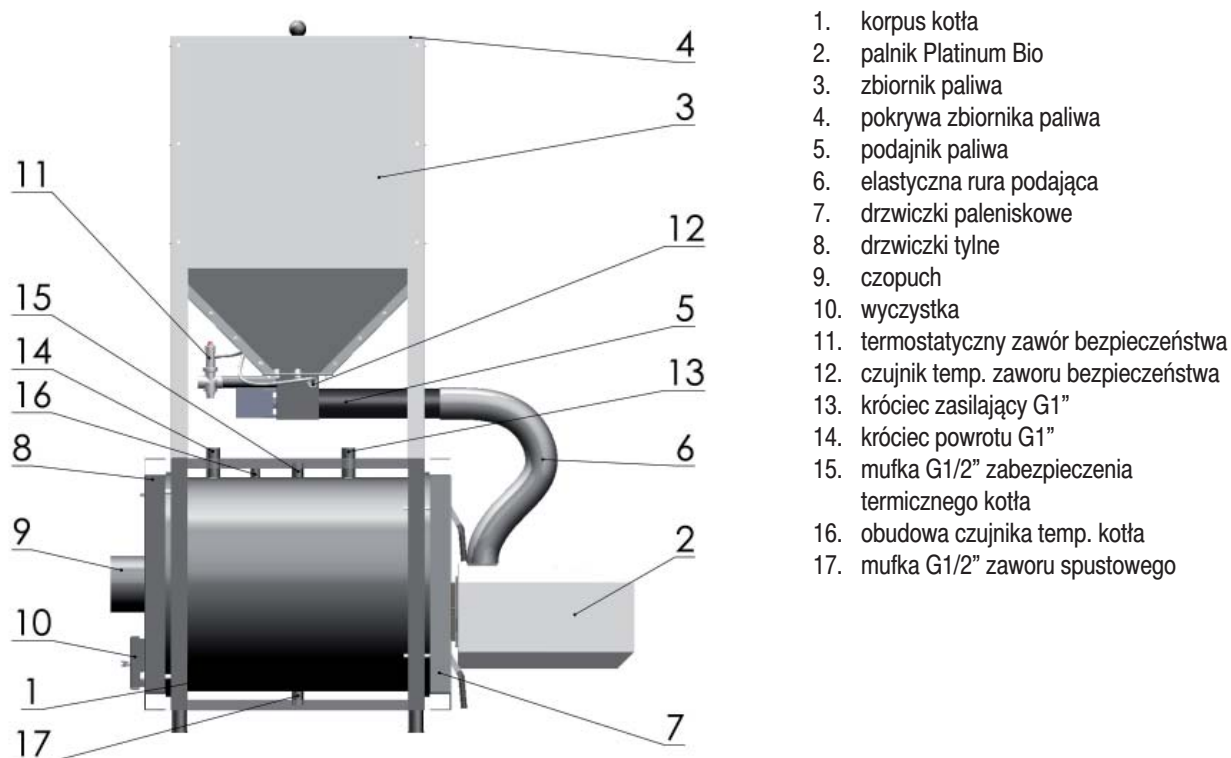
Rys. 01. Podstawowe elementy kotła Mini Bio
